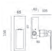
Ref.: GSM03V (tres vías) Grifería empotrada monomando, 3 vías. Laton cromado Box de registro. Cartucho cerámico 35mm
