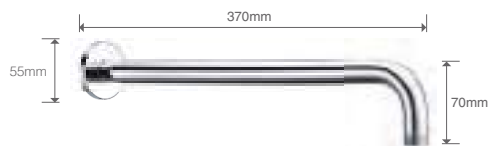
Ref. : BPR001 (latón)
